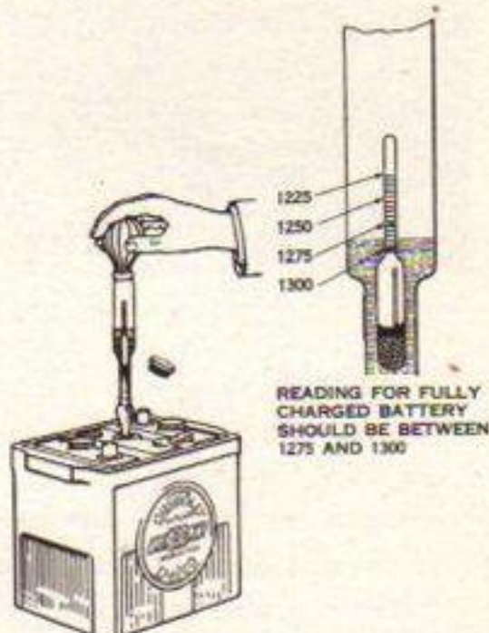
Fig. 32—Hydrometer
