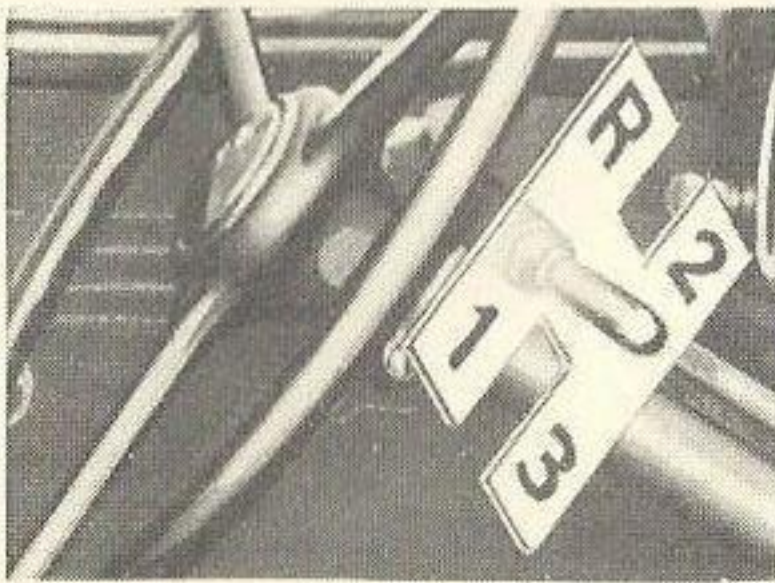
Fig. 17—Gear Shifting
