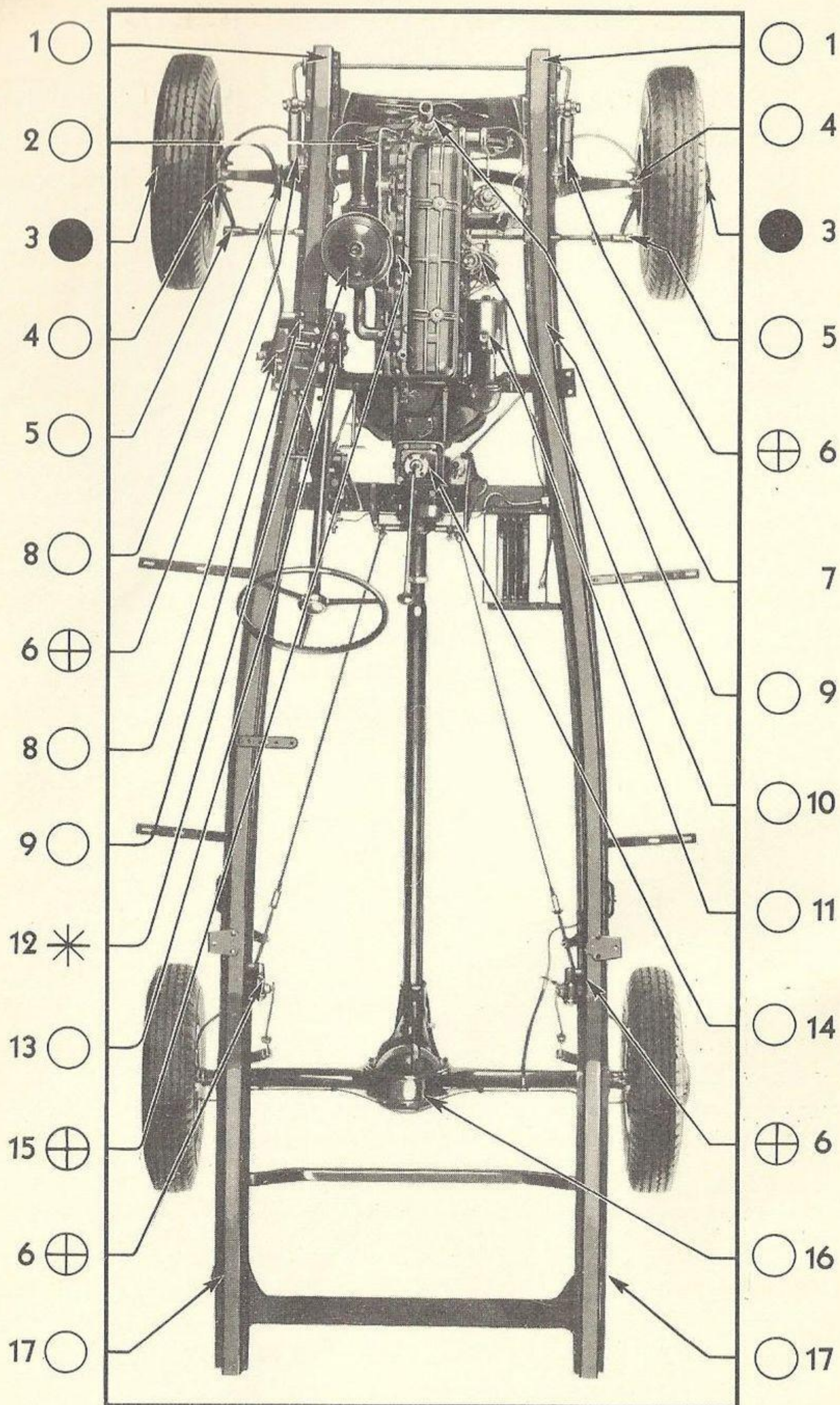
Fig. 38—Master "85"
