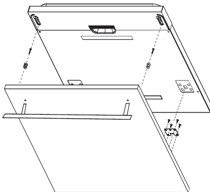
Obrázok 4a Inštalácia krycieho panelu
