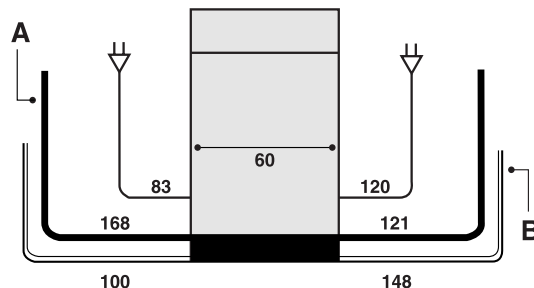
Aansluiting van de buis voor de watertoevoer
